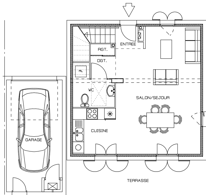
REZ DE CHAUSSEE - 1/100°
